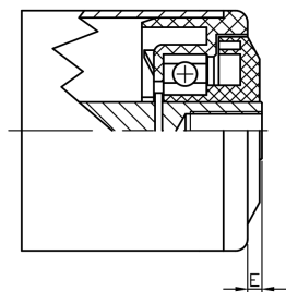
Подшипниковый корпус серии LBA
